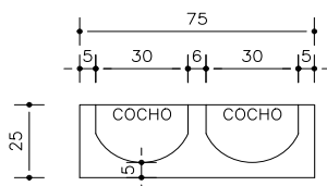
2 CORTE DD DETALHE COCHO ESCALA: 1/25
